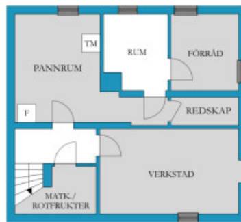
KÄLLARPLAN
